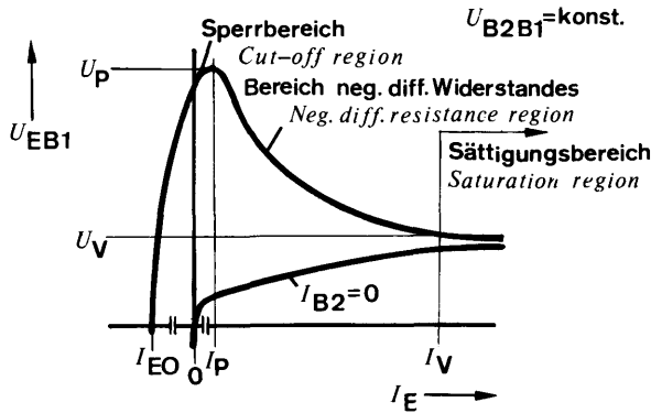
Fig. 1.30. zeigt den Zusammenhang zwischen U_{EB1} und I_E für einen gegebenen Wert von U_{B2B1} sowie für I_{B2} = 0 .
