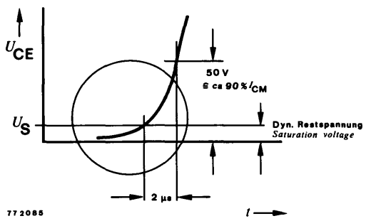
Fig. 1 Definition von U_{Rest\ dyn} Definition from U_{Rest\ dyn}
